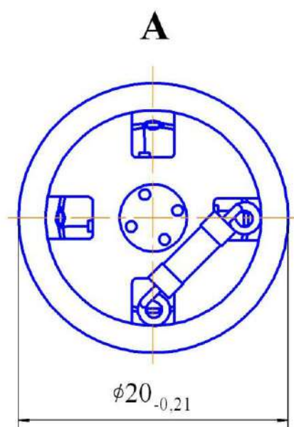
Рисунок Б.3 – DD 2,5; DD 2,5-T
