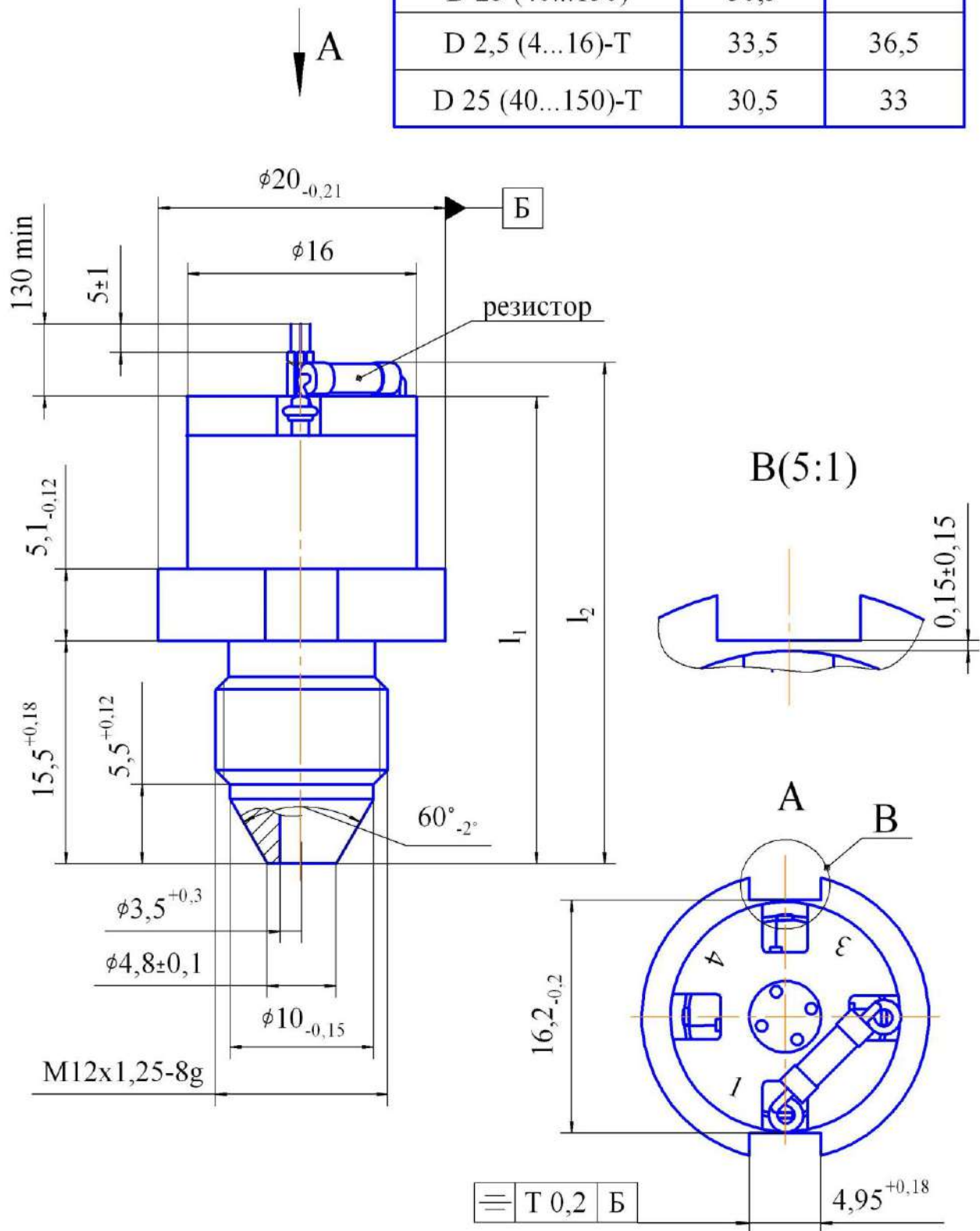
Рисунок Б.2 – D 2,5...D 150; D 2,5-T...D 150-T
